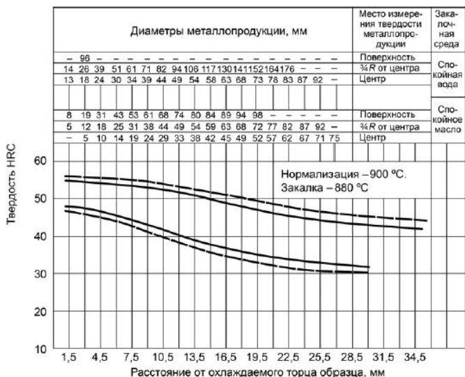
Рисунок А.13 - Сталь марки 38XC
