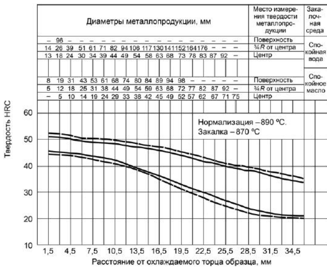
Рисунок А.10 - Сталь марки 27XГР
