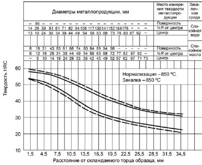
Рисунок А.6 - Сталь марки 45X
