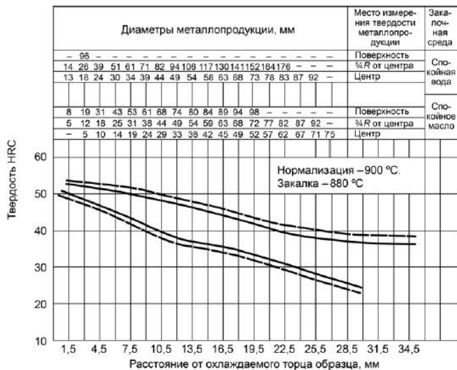
Рисунок А.18 - Сталь марки 30ХГСА
