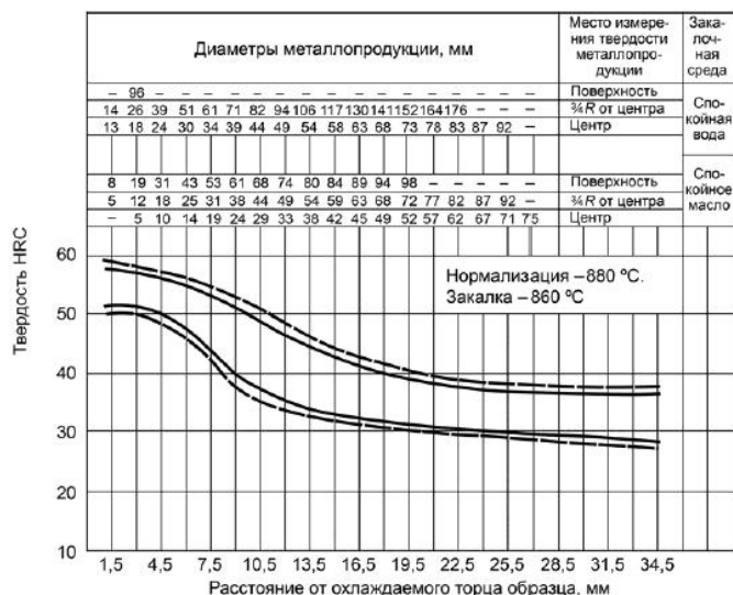
Рисунок А.14 - Сталь марки 40XФА
