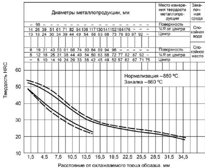
Рисунок А.3 - Сталь марки 30X
