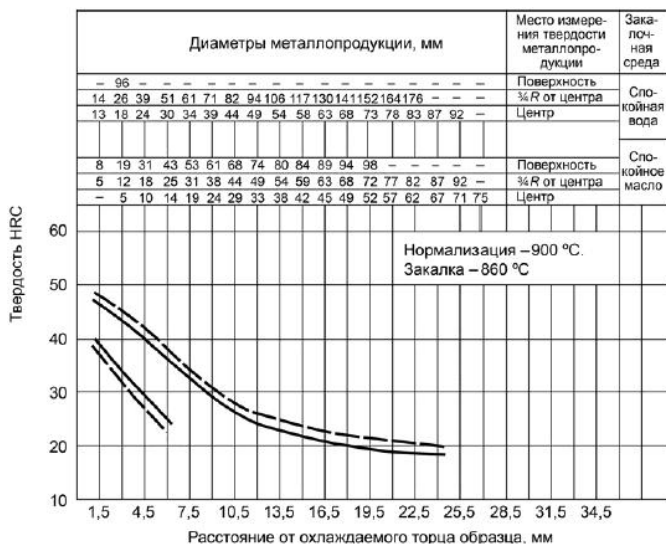
Рисунок А.2 - Сталь марки 20X
