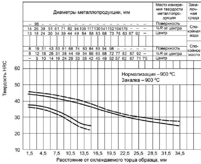
Рисунок А.9 - Сталь марки 20XГР
