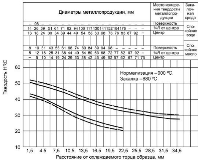
Рисунок А.8 - Сталь марки 30XГТ
