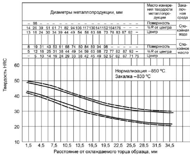
Рисунок А.16 - Сталь марки 20ХН3А
